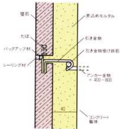
帯とろ工法の例
