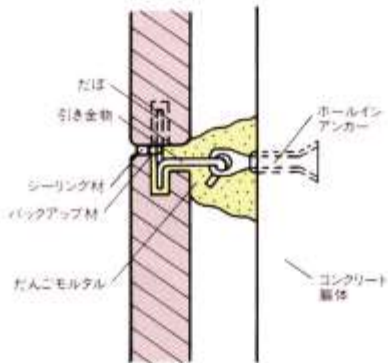
空積み工法の例
