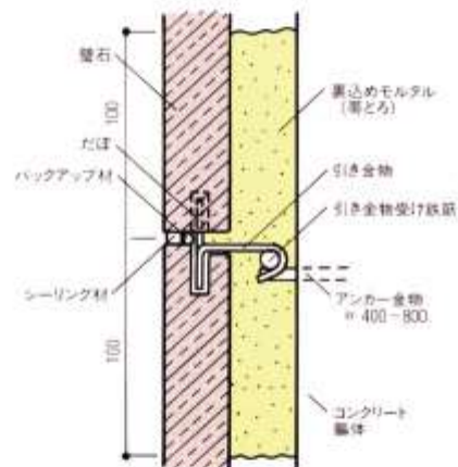
帯とろ工法の例
