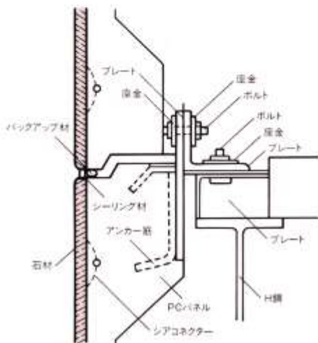
PCパネル石打込み工法の例
