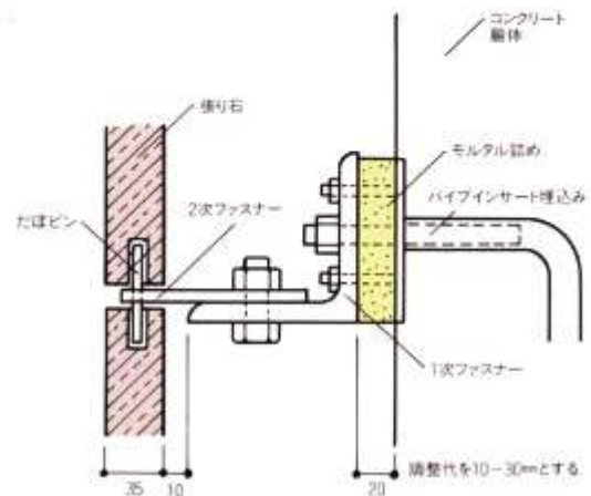
乾式石張り工法の例
